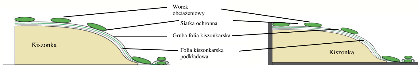
Schemat 3 : przekrój podłużny Silos pryzma / Silos korytarz
